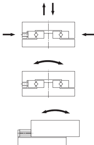
图2 负荷方向
