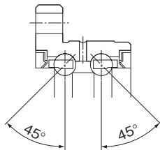
图2 BNS-V型、BNS-A型支撑轴承的结构
