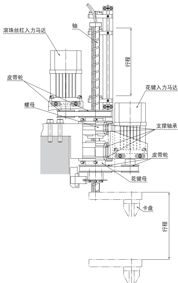
图5 BNS型的使用例
