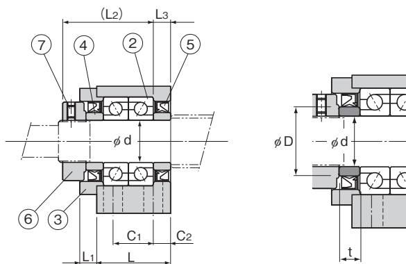
套环详情
