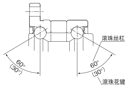
图1 BNS型支撑轴承的结构
