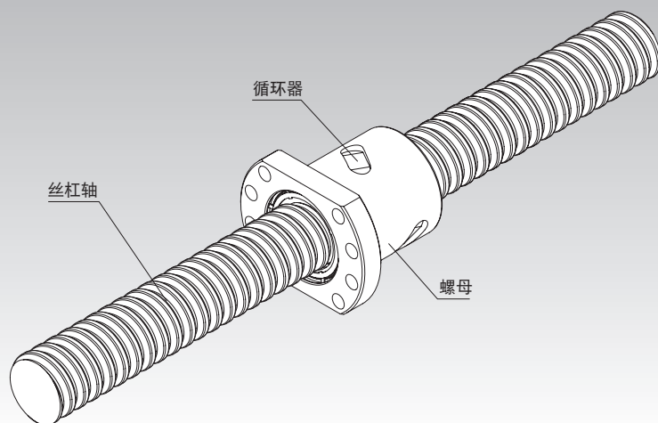
图1 符合ISO3408标准滚珠丝杠
