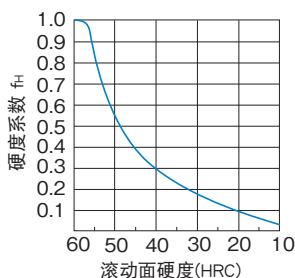
图1 硬度系数( f_H )
