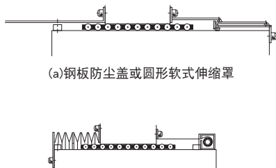
(a)钢板防尘盖或圆形软式伸缩罩 (b)伸缩防尘罩或卷帘 图1 防尘方法
