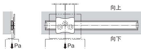
图10 适合E36RS型
