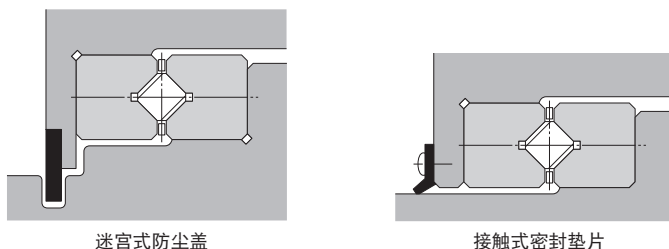
图2 防尘方法
